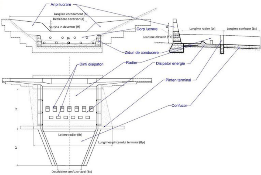
Metodologie de urmărire în timp a lucrărilor transversale de corectare a torențiilor și de eşalonare a intervențiilor cu lucrări de reparații
