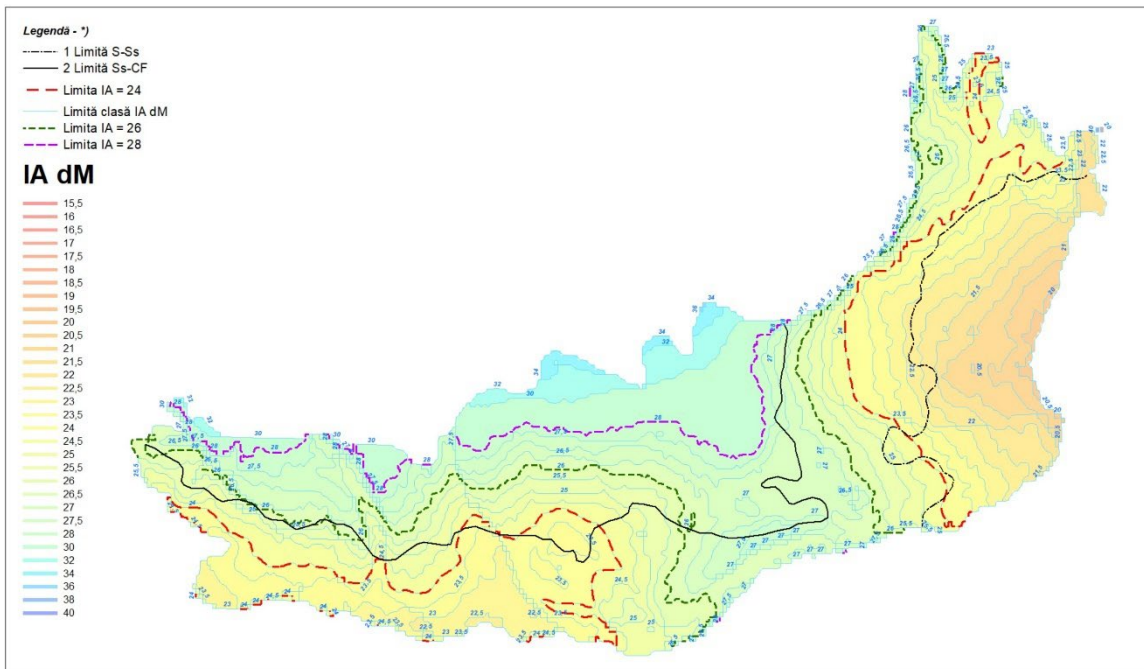
Indicele de ariditate de Martonne - Perioada 1991-2020
